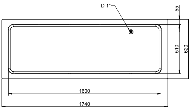
Boven aanzicht
